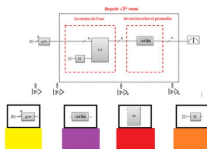
Figura 56. Diagrama del algoritmo cuántico de Grover nivel 1- reto 2
