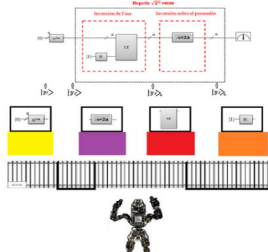
Figura 57. Referencia resolución reto del diagrama algoritmo cuántico de Grover nivel 1- reto 2
