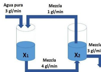
Figura 12. Dos tanques mezcladores
