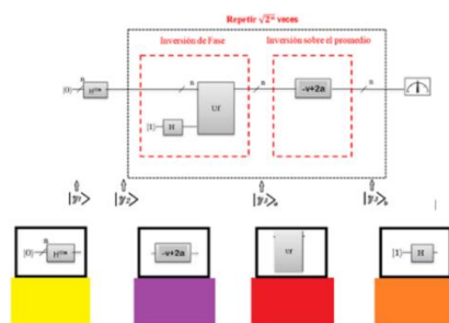
Figura 56. Diagrama del algoritmo cuántico de Grover nivel 1- reto 2
